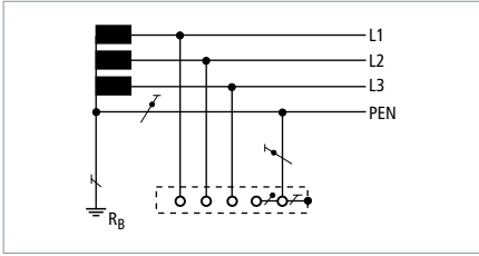
Système TN-C 230 / 400 V
