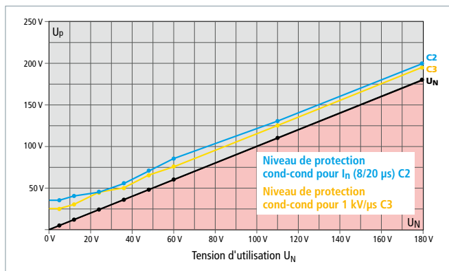
Diagramme du niveau de protection BXTU
