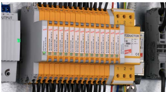
BLITZDUCTORconnect pour la protection des systèmes de mesure et de contrôle
