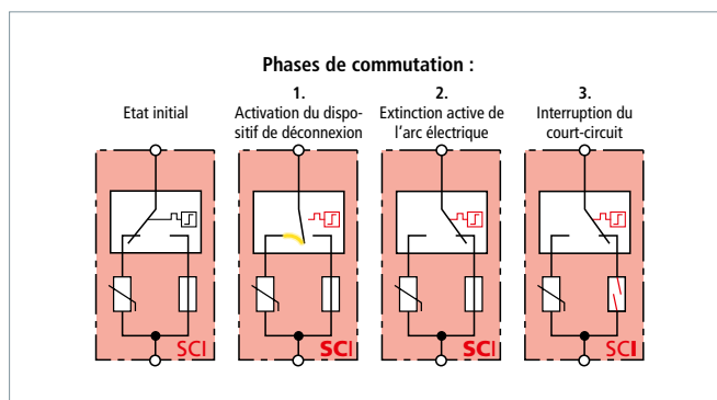
Dispositif de commutation DC à trois étapes (principe breveté SCI)
