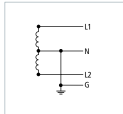
1 phase; 4 conducteurs actifs Phases 'éclatées' ou Edison (1 Ph, 3 fils + G) 120 V / 240 V
