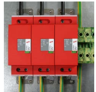
Montage flexible à l'aide d'un étrier de montage
