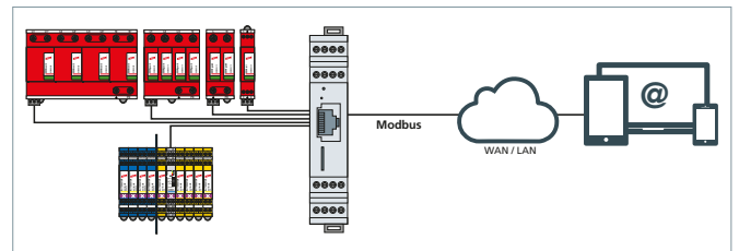
Construction du système global d'alerte DEHNrecord avec des parafoudres Red / Line et Yellow / Line.
