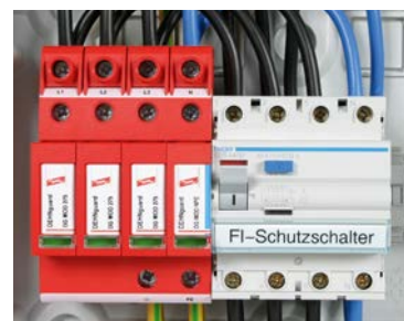
Réalisation d'un câblage en V selon la norme NF C15-100 grâce au bornier STAK 2X16.
