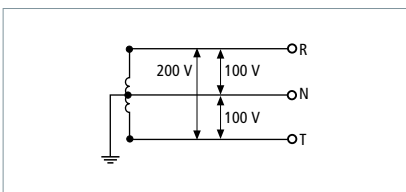
2 phases; 3 conducteurs actifs (1 Ph, 3 fils) 100 V / 200 V
