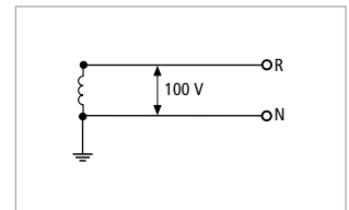
1 phase; 2 conducteurs actifs (1 Ph, 2 fils) 100 V
