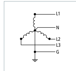
3 phases; 5 conducteurs actifs (3 Ph Y, 4 fils + G) 120 V / 208 V 277 V / 480 V
