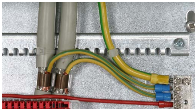
Système de connexion particulièrement peu encombrant sous la forme d'un ressort de contact. Compensation du fluage des matériaux du câble grâce à la pression du ressort.
