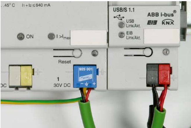
Protection d'un bloc d'alimentation KNX avec le BUSector. Montage dans l'emplacement de réception du terminal de bus standard.
